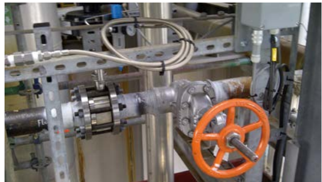
Abb. 6 Das neue Gleitschieberventil mit 8049 Stellungsregler.
